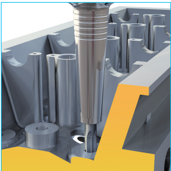
Reiben in engen Bearbeitungsräumen Reaming in tight space
